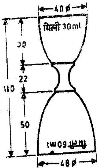
60 मिमी और 30 मिमी चारिता के मिश्रित निकर माप के आकार तथा अभिहित विमा आकृति - १८
