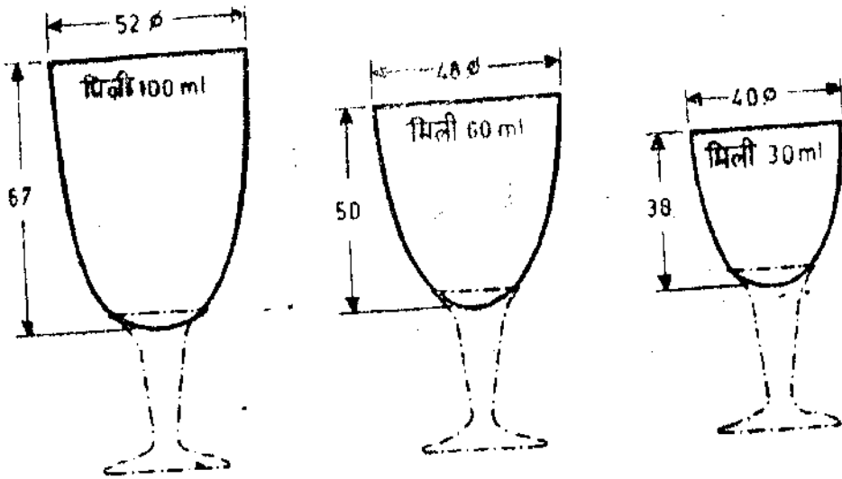
निकर माप के आकार तथा विमा 100 मिमी, 60 मिमी और 30 मिमी आकृति - १७
