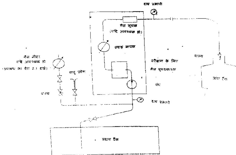
चित्र २- वाहन परीक्षण में गैस पंचायक के लिए सुविधा
