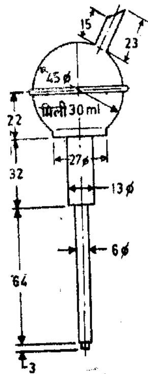
30 मिमी चारिता के स्वचालित निकर माप के आकार तथा अभिहित विमा आकृति - १९
