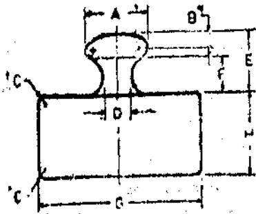
पुडो करेट के बाट भाकृति - १० (10)
